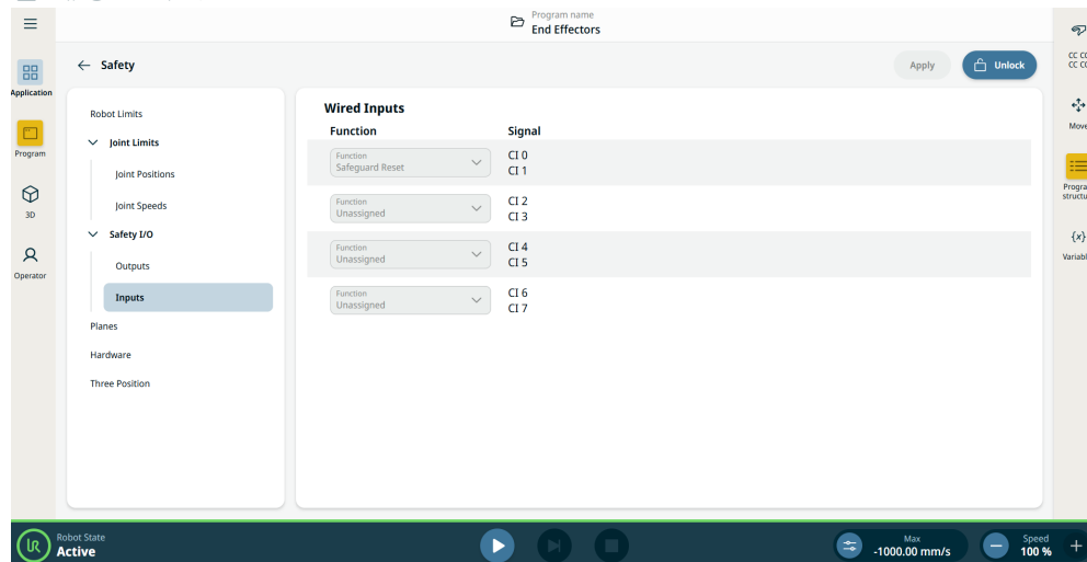
그림 1.4: 입력 신호를 표시하는 PolyScope X 화면.
