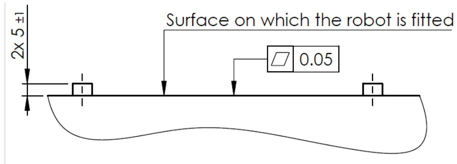
1.2: 로봇 베이스용 장착 플레이트
