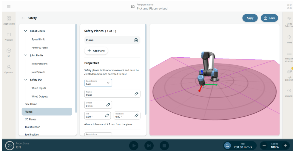
그림 1.5: 안전 플레인을 표시하는 PolyScope X 화면.
