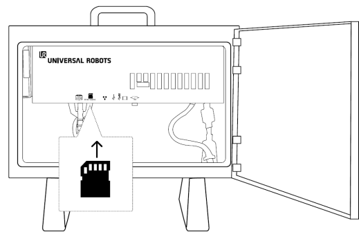
컨트롤 박스
